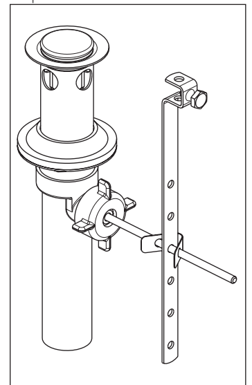
RP38958▲ 50/50 Pop-Up Assembly Less Lift Rod Ensamble del Desagüe Automático sin la barra para alzarlo Renvoi mécanique sans la tirette
